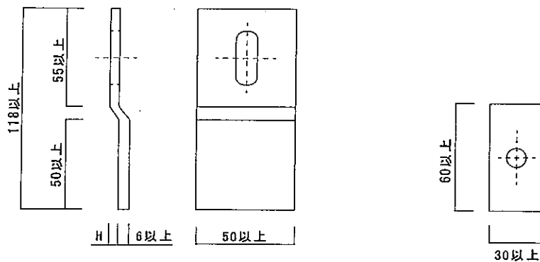
角ナット
