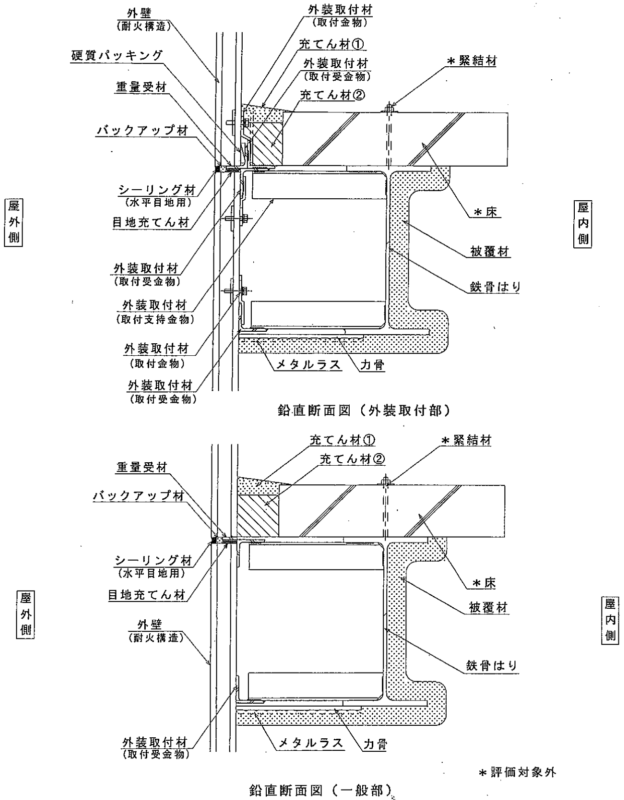
図2 構造説明図
