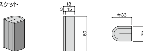
端部ガスケット A
