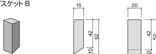
端部ガスケット B
