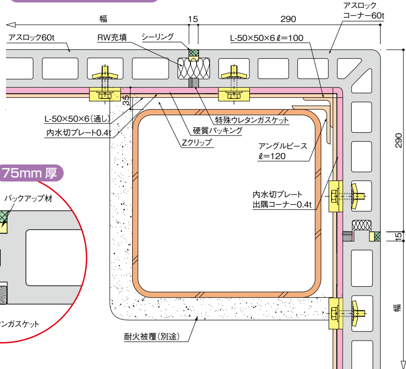
出隅コーナー部水平断面
