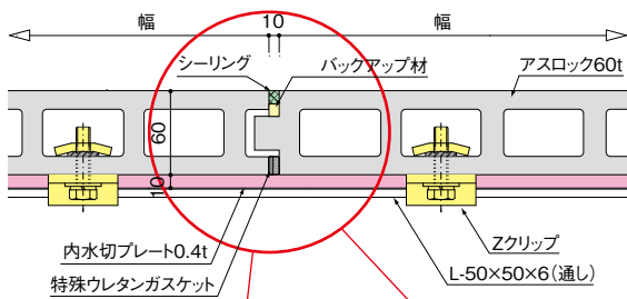
一般部水平断面
