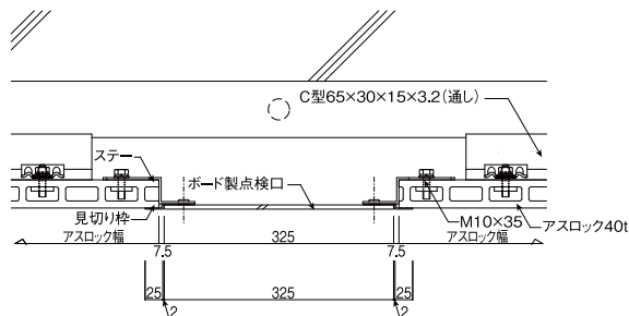
A-A'断面図
