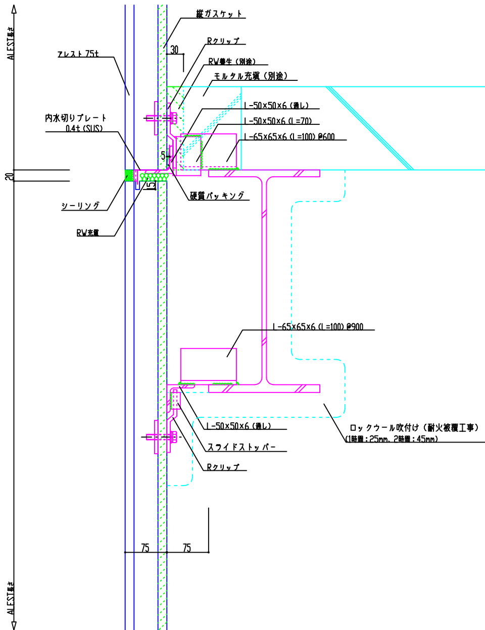
縦断面詳細図
