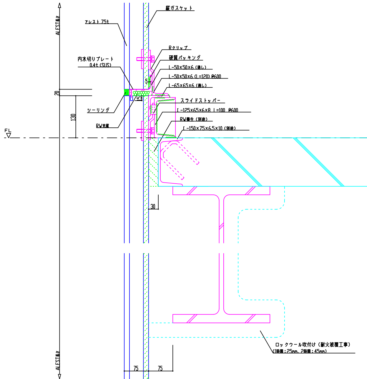
縦断面詳細図 (梁せい大)
