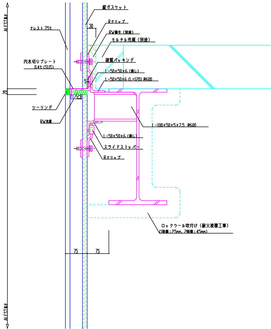
縦断面詳細図
