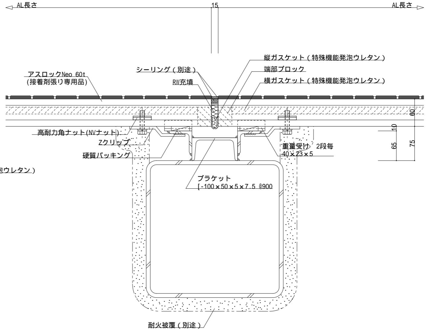
水平断面詳細図
