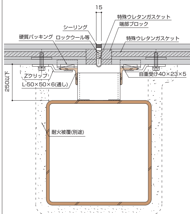
図31 縦目地部
