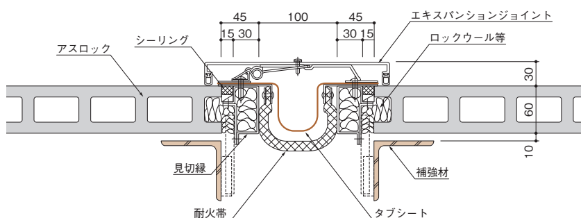
図73 エキスパンションジョイント金物の取付け（縦張り工法）
