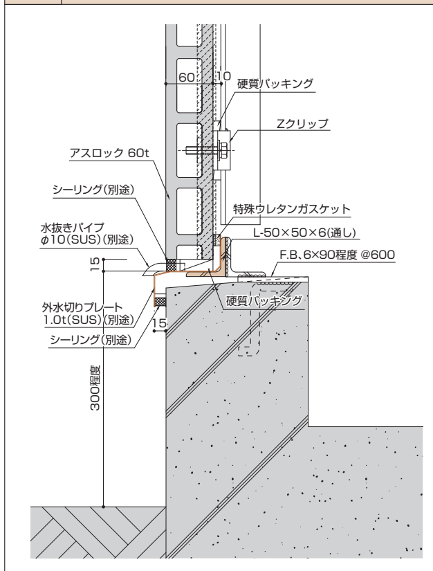
図36 下部（一体形外水切）
