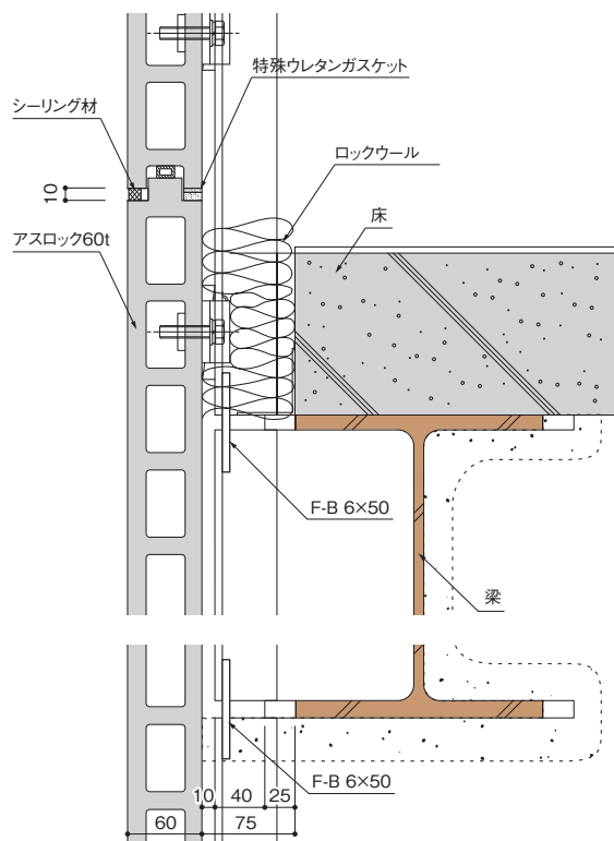
図35 縦目地部（梁部）
