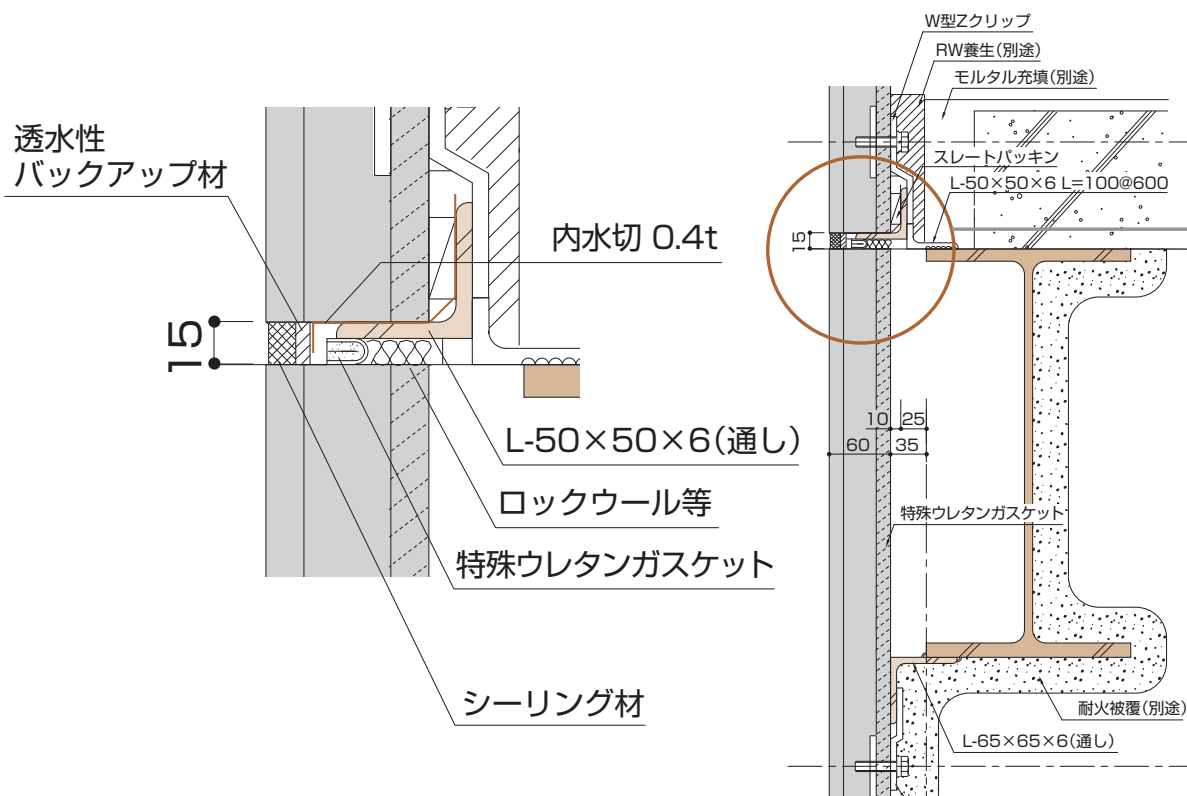
図30 横目地部
