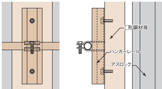
図67 片サドル
