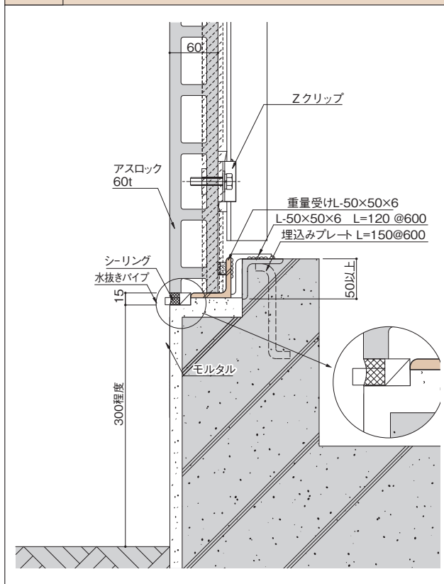
図38 下部（水切無し）
