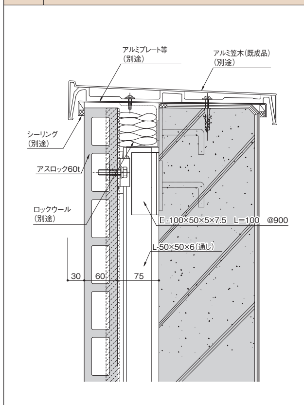
図40 上部（オープン笠木）
