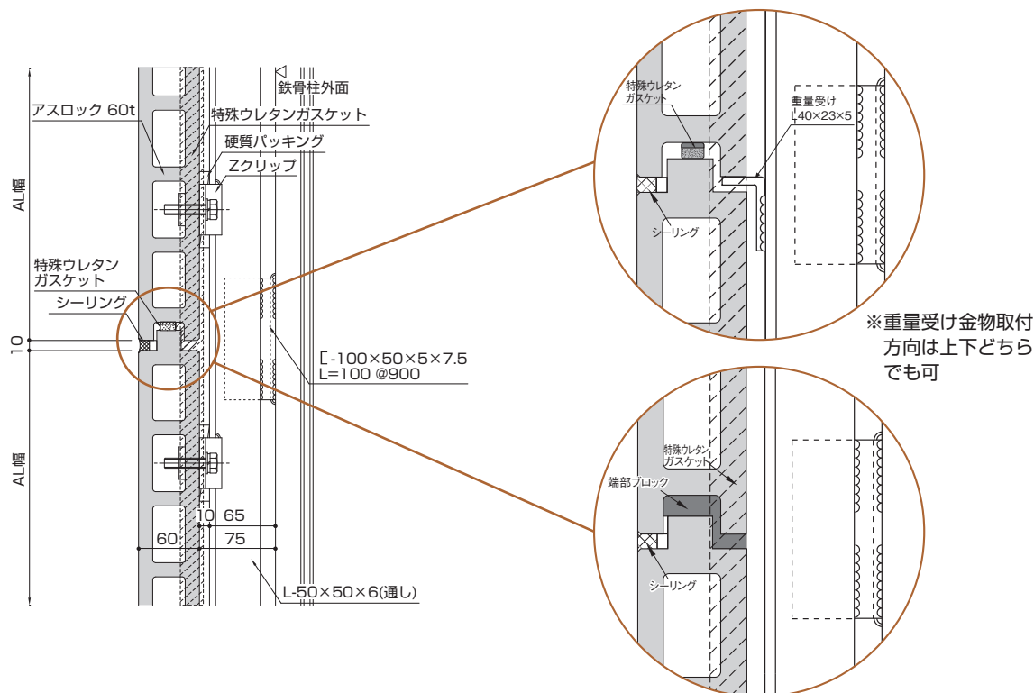
図34 横目地部（一般部）
