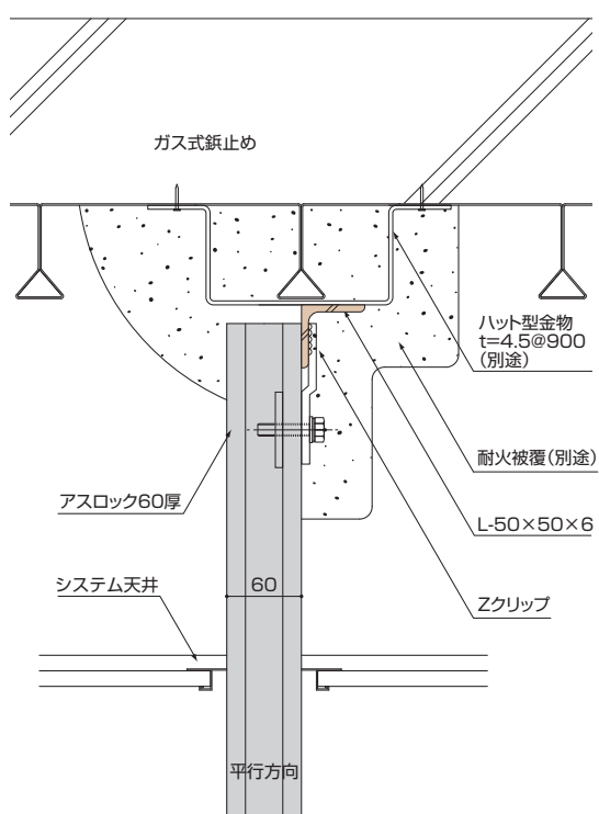
図54 上部（フラットデッキ平行方向）
