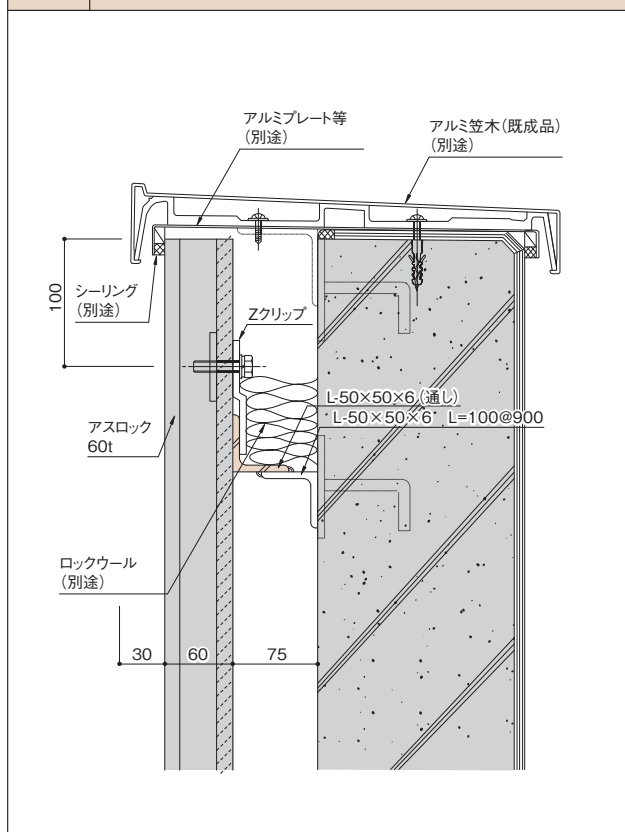
図12 上部（オープン笠木）
