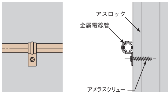
図67 片サドル
