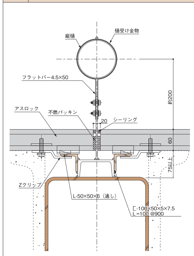
図70 樋の取付け（横張り工法）
