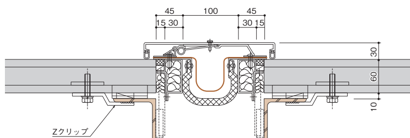
図74 エキスパンションジョイント金物の取付け（縦張り工法）
