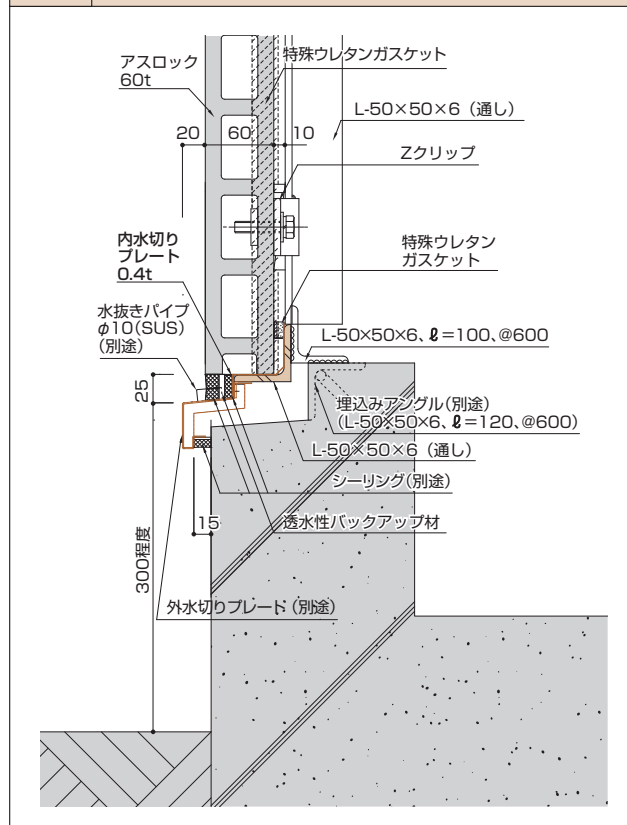
図37 下部（組み合せ水切）
