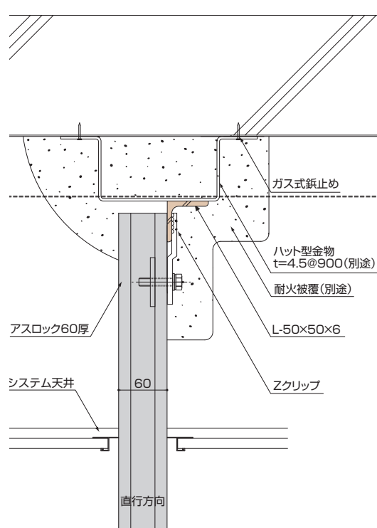
図55 上部（フラットデッキ直行方向）
