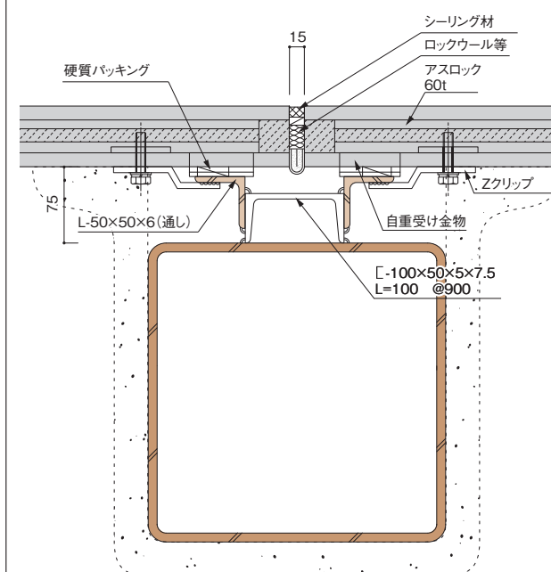
図33 縦目地部
