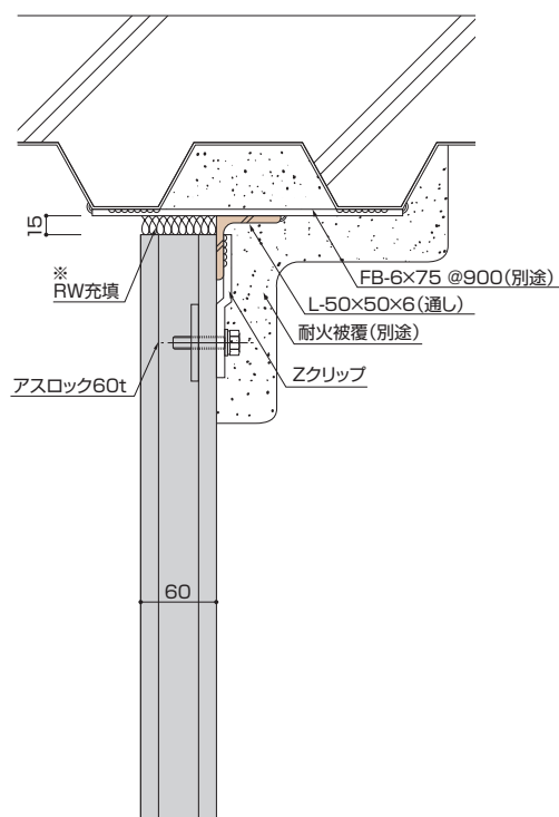
図52 上部（デッキプレート）
