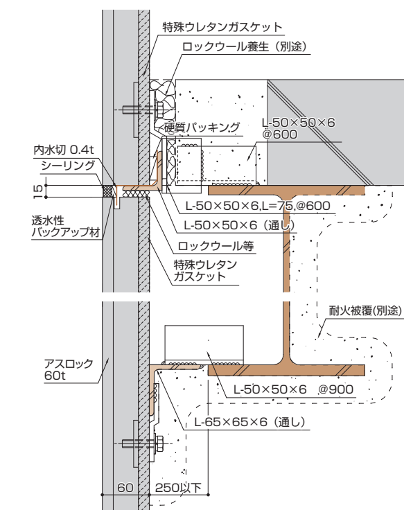
図5 横目地部 (クリアランス60~250mm)
