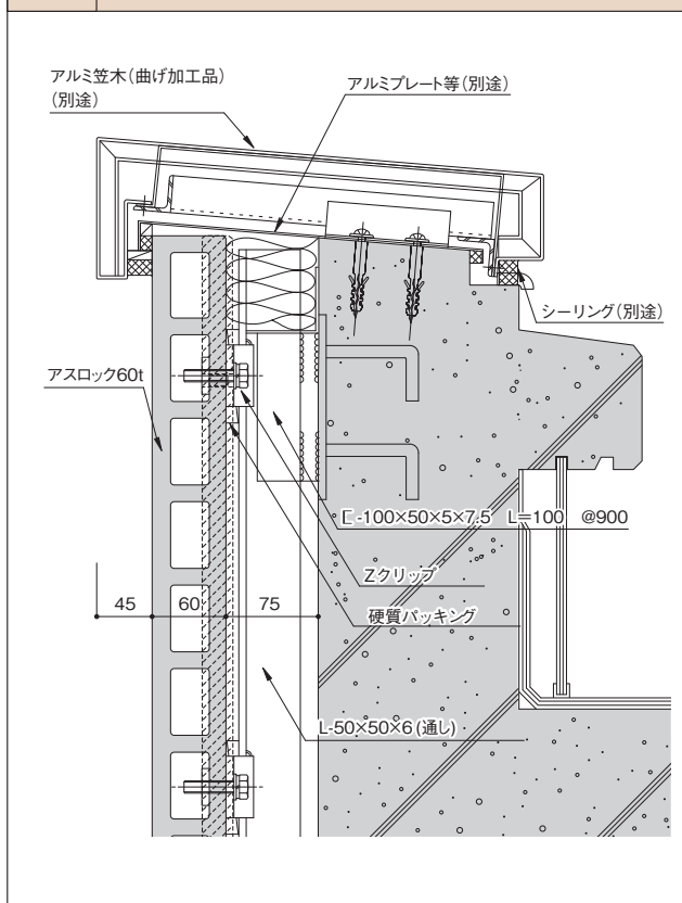
図39 上部（クローズ笠木②）
