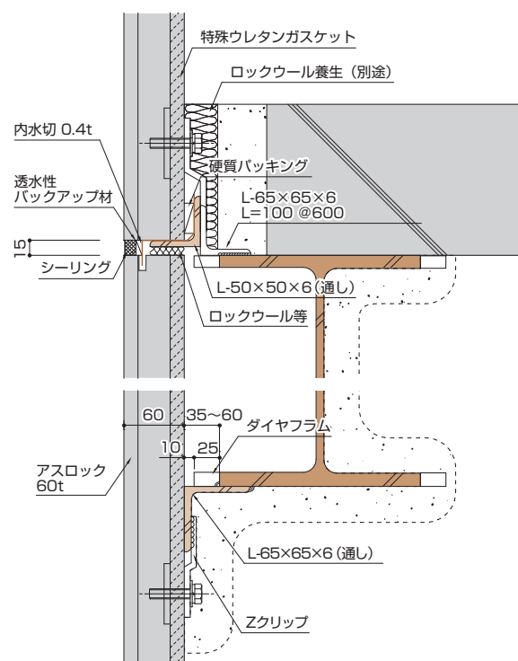
図4 横目地部 (クリアランス35~60mm)
