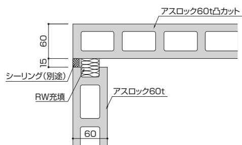
図61 壁付部
