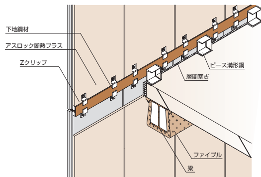
〔縦張り工法〕
