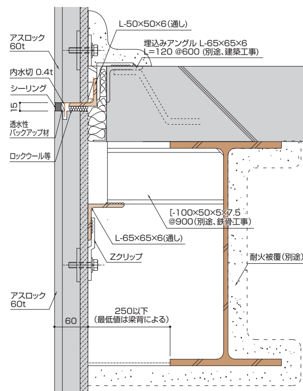
図7 横目地部 (クリアランス60~250mm、スラブ固定)
