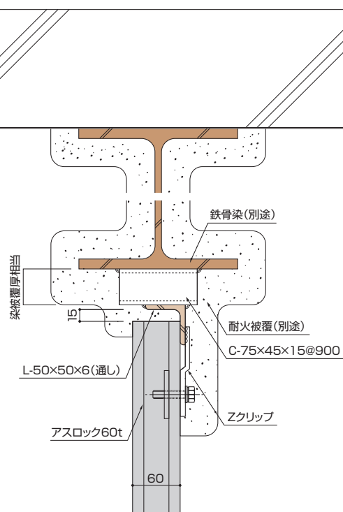
図53 上部（梁）
