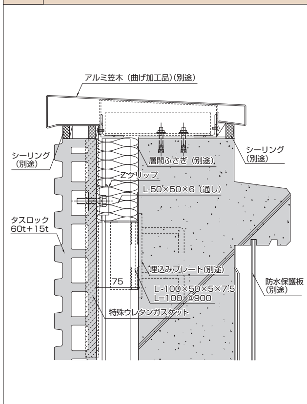
図41 上部（デザインパネル使用時）
