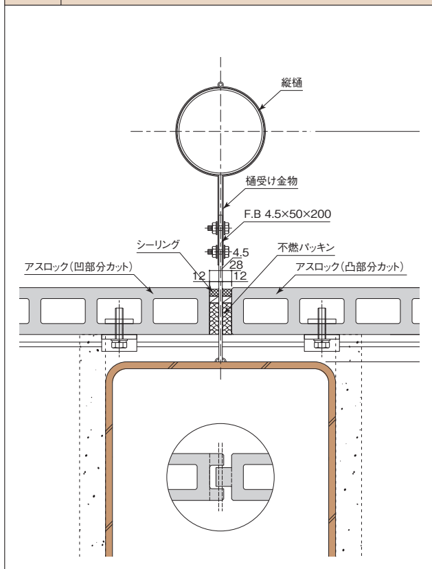
図69 樋の取付け（縦張り工法）
