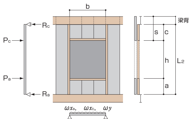
標準方式
