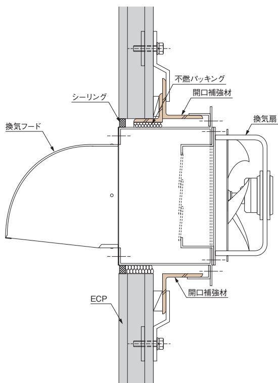
図63 換気扇（縦断面）
