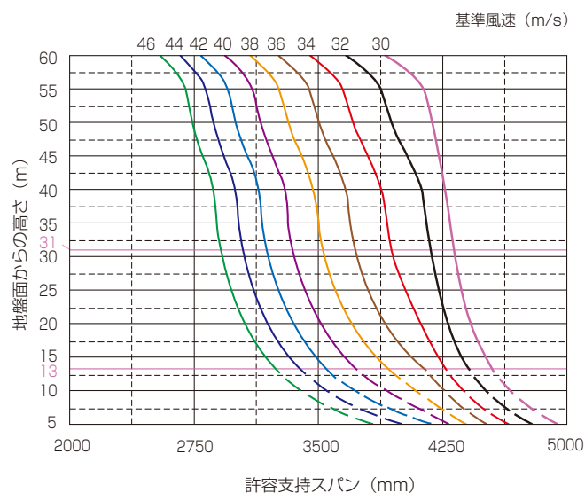
アスロック 60mm厚フラット品（再現期間100年）
