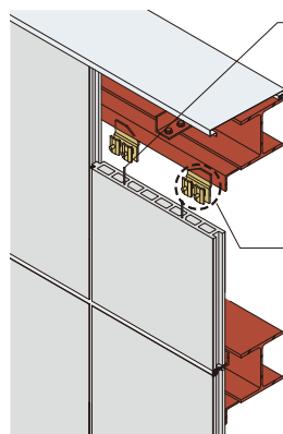
縦張り工法
