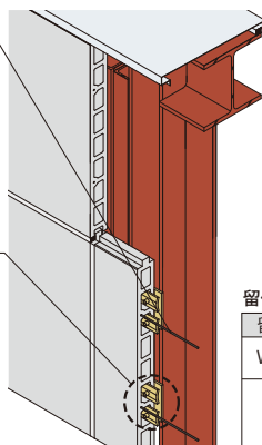
横張り工法
