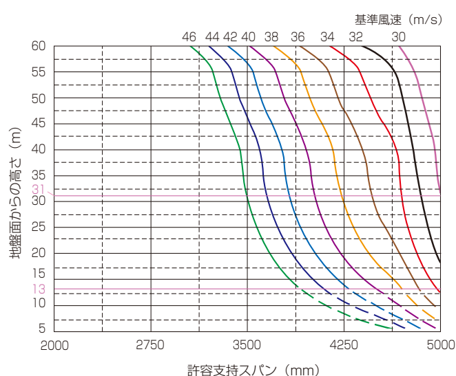
アスロック 75mm厚フラット品（再現期間100年）
