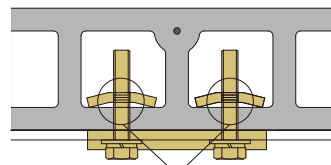
留付金具の種類と設計許容耐力値
