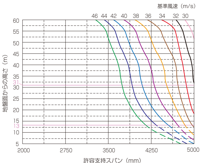
アスロック 75mm厚フラット品（再現期間50年）
