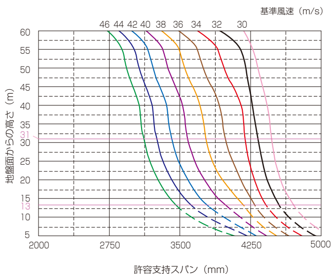
アスロック 60mm厚フラット品（再現期間50年）
