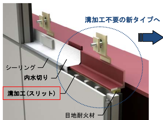
既存ニューセフティ縦張り工法
