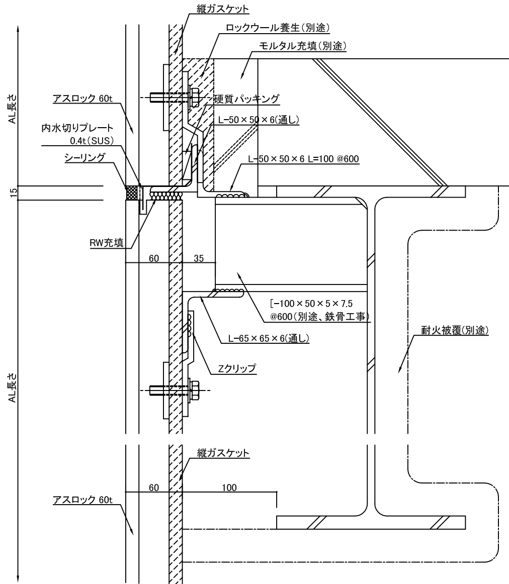
アスロック垂直断面図 (100mmクリアランス・梁上部固定)
