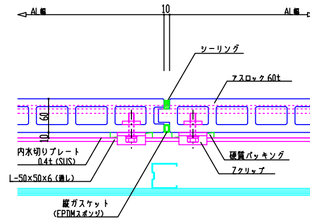
水平断面図
